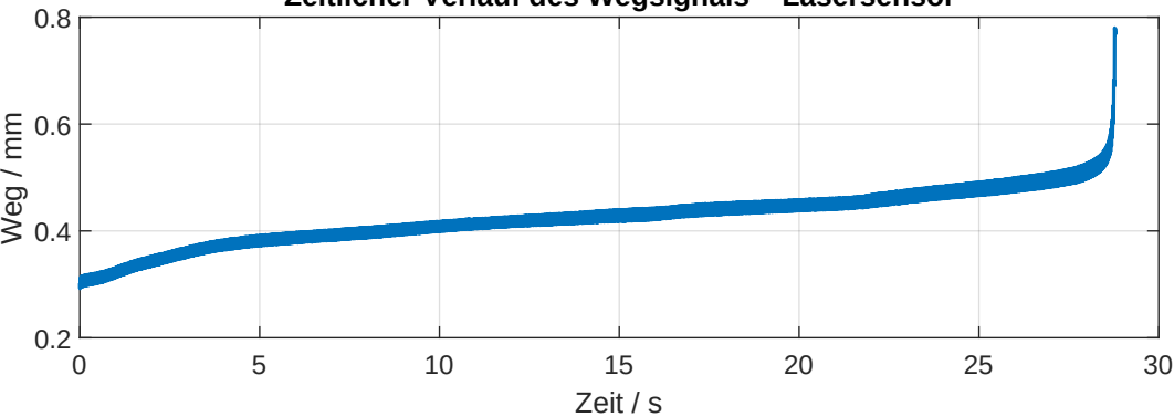
Zeitlicher Verlauf des Wegsignals – Lasersensor
